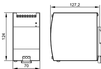
Рисунок / Figure / Сурет 6 – Габаритные размеры / Overall dimensions / Ушығ габариттік өлшемдері OPSE-DC24-480B
