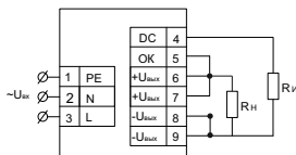
Рисунок / Figure / Сурет 10 – Схема подключения / Connection diagram / Жалғау схемасы OPSE-DC24-240B (RL – нагрузка индикации / load indicator / индикация жүктемесі)
