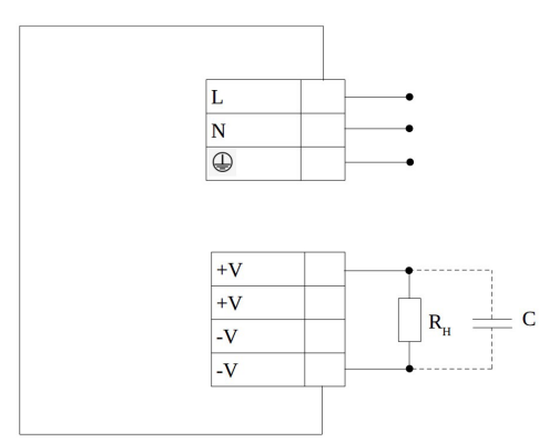
Рис. 1 Схема подключения блока питания
