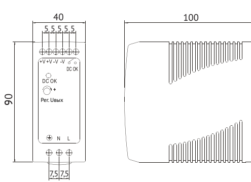
Рис.3 Габаритные размеры блоков питания MDR-40, 60
