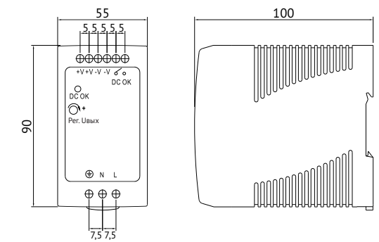
Рис.4 Габаритные размеры блоков питания MDR-100
