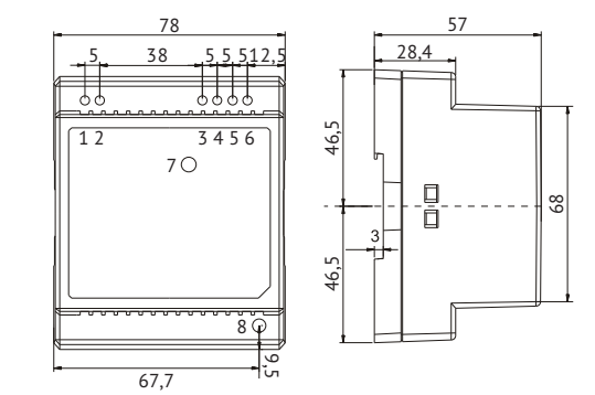
Рис.5 Габаритные размеры блоков питания DR-15
