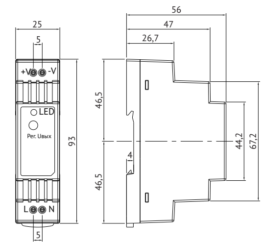
Рис.5 Габаритные размеры блоков питания DR-15
