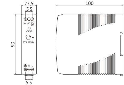
Рис.2 Габаритные размеры блоков питания MDR-10, 20
