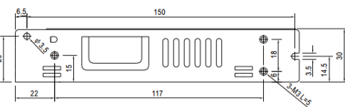
Рисунок А.4 – Габаритные размеры блоков питания LRS-150
