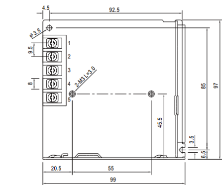
Рисунок А.1 – Габаритные размеры блоков питания LRS-35; LRS-50; LRS-60
