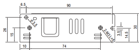
Рисунок А.2 – Габаритные размеры блоков питания LRS-75
