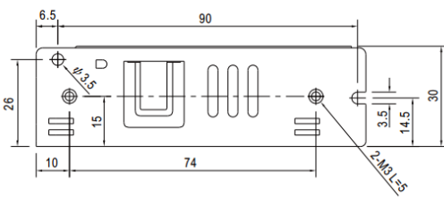
Рисунок А.1 – Габаритные размеры блоков питания LRS-35; LRS-50; LRS-60
