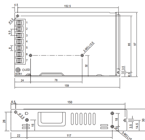
Рисунок А.4 – Габаритные размеры блоков питания LRS-150
