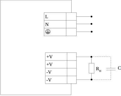
Рисунок 1 - Схема подключения блока питания
