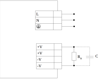
Рисунок 1 - Схема подключения блока питания
