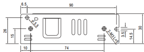
Рисунок А.2 – Габаритные размеры блоков питания LRS-75
