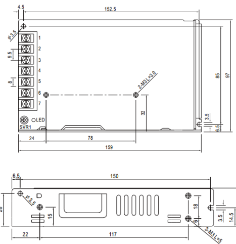
Рисунок А.4 – Габаритные размеры блоков питания LRS-150
