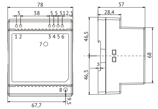
Рис.5 Габаритные размеры блоков питания DR-15
