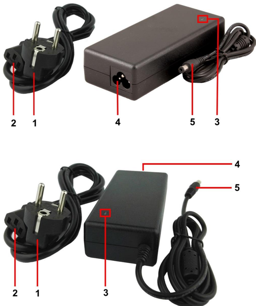
Рис. 1 Блоки питания PS-48065, PS-48096, PS-48135, внешний вид, разъемы и индикаторы
