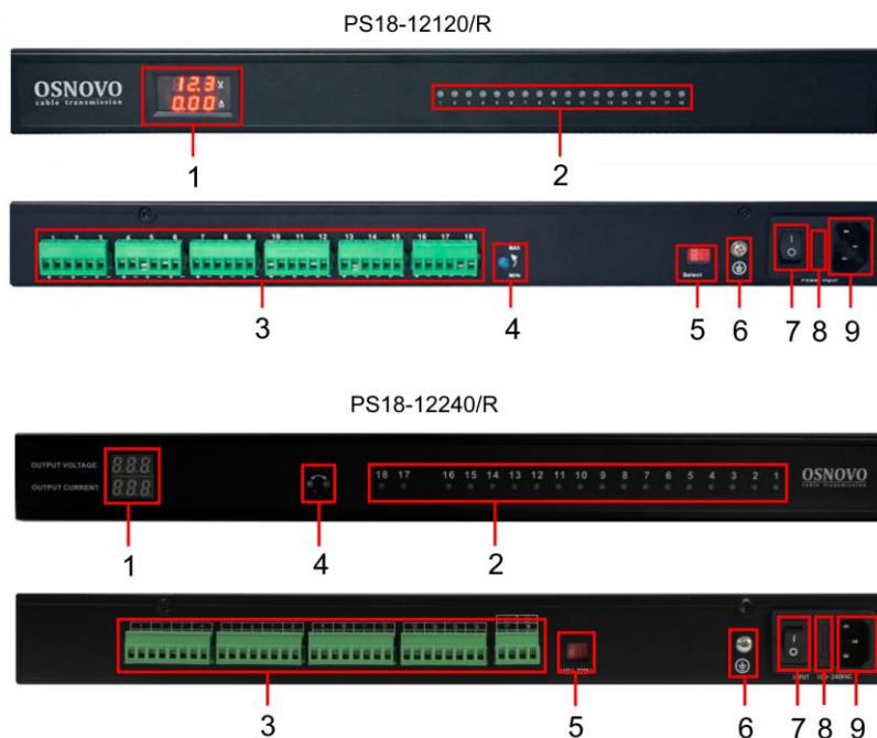
Рис.2 Блоки питания PS18-12120/R, PS18-12240/R, разъемы и индикаторы передней и задней панелей
