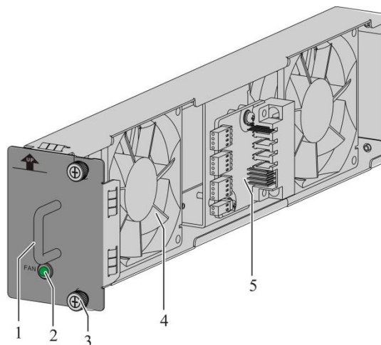
Рисунок 1-9. Модуль QSR-M-3920-FAN
