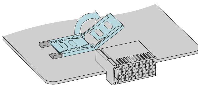
Рисунок 3-9. Переверните защелку
