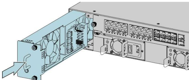
Рисунок 6-12. Вставьте модуль вентиляторов в шасси
