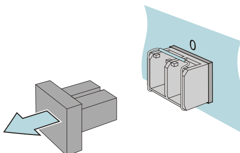
Рисунок 6-16. Снимите пылезащитную крышку модуля SFP
