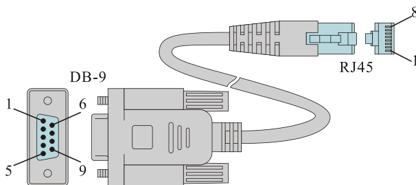
Рисунок 4-1. Консольный кабель
