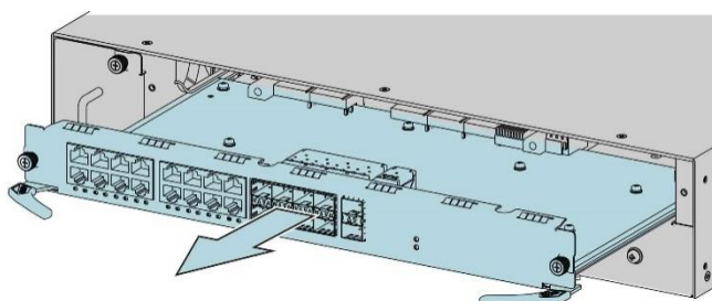
Рисунок 6-5. Вытащите 3ESP, шаг 3
