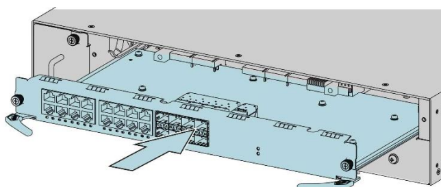
Рисунок 6-6. Вставка 3ESP.
