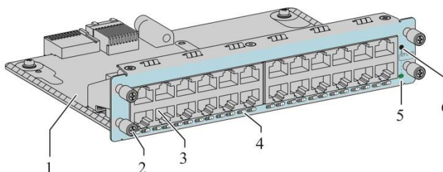
Рисунок 1-5. Внешний вид карты серии M-3920
