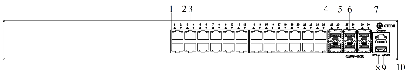
Рисунок 1-3. Передняя панель QSW-4530-30TX
