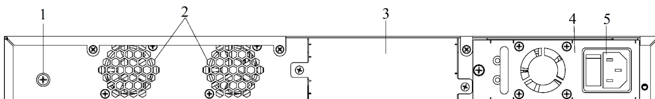
Рисунок 1-4. Задняя панель QSW-4530-30TX
