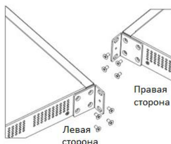
Рисунок 3-1. Присоединение крепежных кронштейнов к коммутатору
