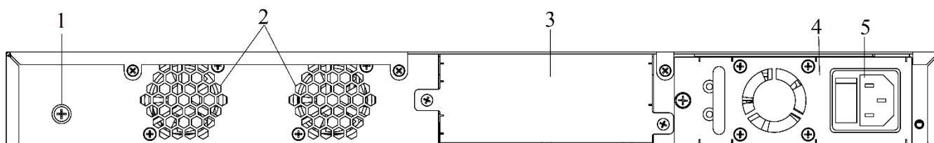
Рисунок 1-8. Задняя панель QSW-4530-54TX
