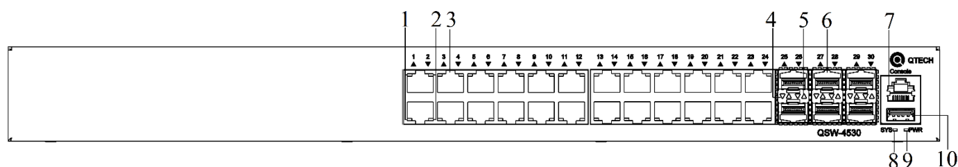
Рисунок 1-1. Передняя панель QSW-4530-30TX-POE
