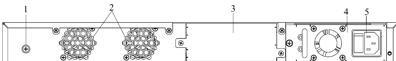
Рисунок 1-6. Задняя панель QSW-4530-54TX-POE
