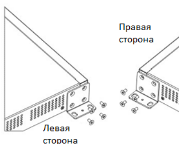
Рисунок 3-2. Присоединение крепежных кронштейнов к коммутатору для установки на стену
