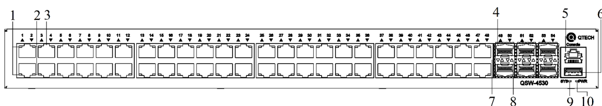
Рисунок 1-7. Передняя панель QSW-4530-54TX
