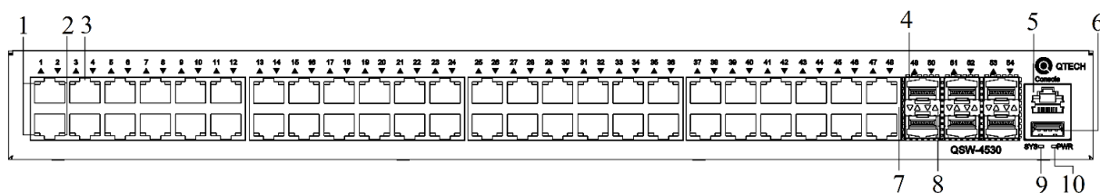
Рисунок 1-5. Передняя панель QSW-4530-54TX-POE
