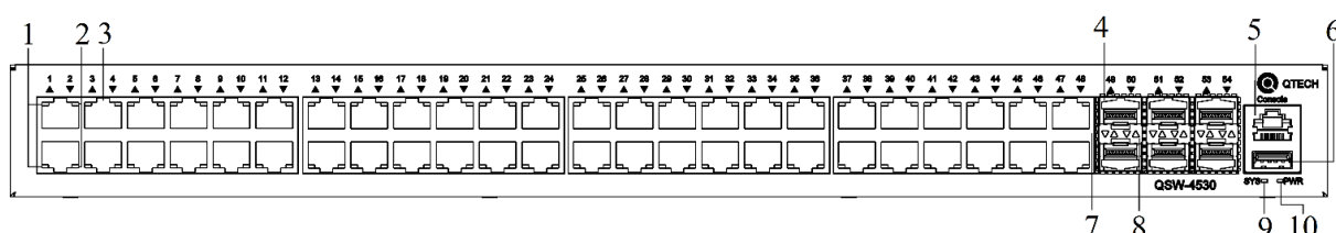
Рисунок 1-7. Передняя панель QSW-4530-54TX
