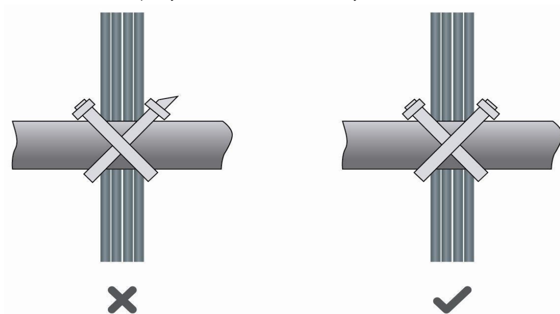
Рисунок 8-2. Стяжка проводов (2)
