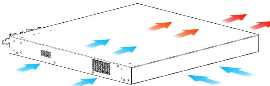
Рисунок 1-4. Направление потоков воздуха
