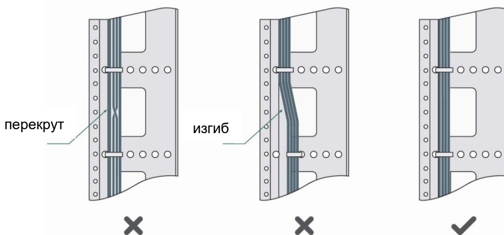
Рисунок 7-4. Прикрепление кабелей
