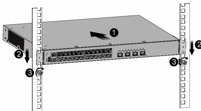
Рисунок 3-3. Затяжка винтов
