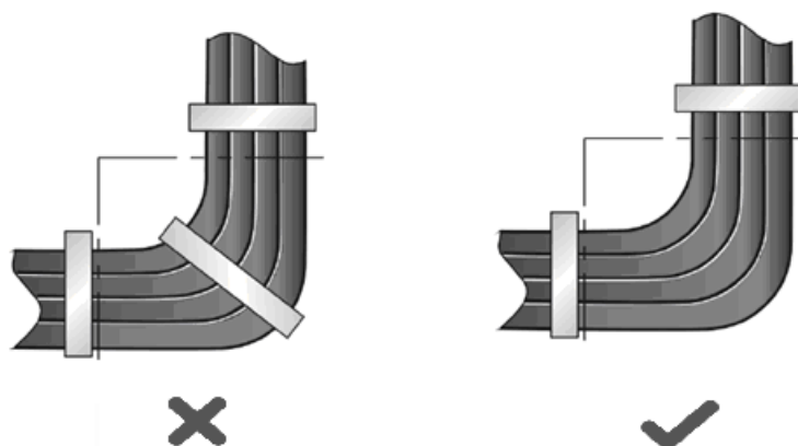
Рисунок 7-6. Стяжка кабелей
