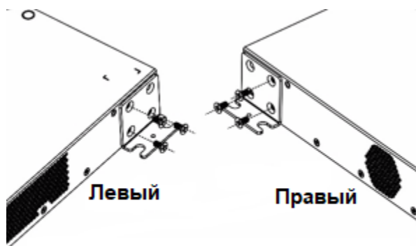
Рисунок 3-5. Закрепление кронштейнов
