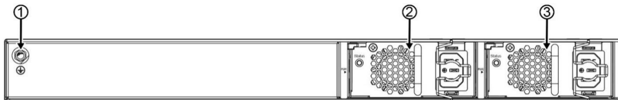
Рисунок 1-15. Задняя панель QSW-4700-52TX-POE
