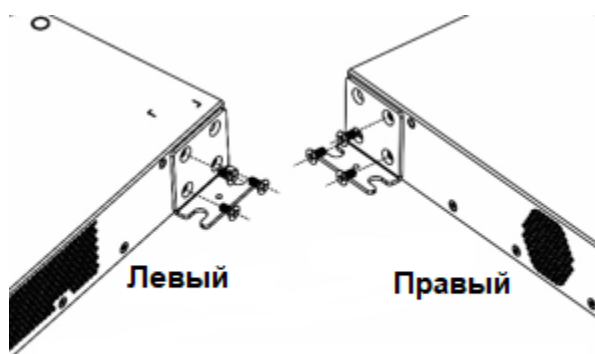
Рисунок 3-5. Закрепление кронштейнов
