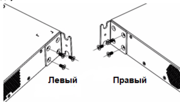
Рисунок 3-1. Монтаж кронштейнов на коммутатор
