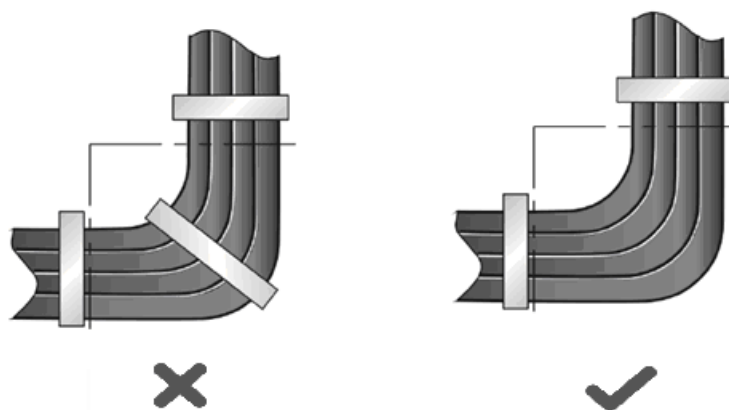
Рисунок 7-6. Стяжка кабелей
