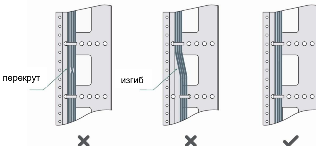
Рисунок 7-4. Прикрепление кабелей
