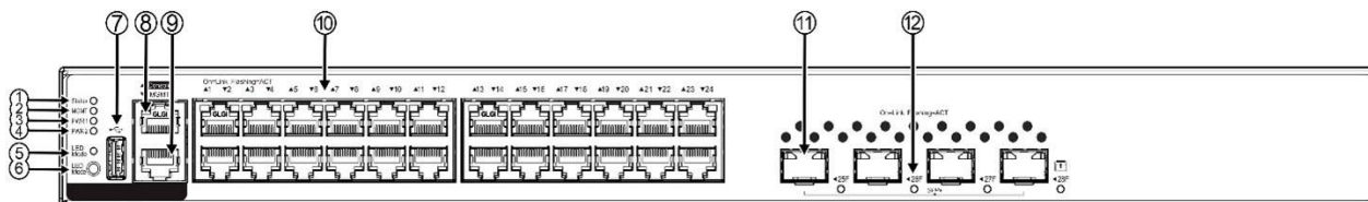
Рисунок 1-10. Передняя панель QSW-4700-28TX-POE
