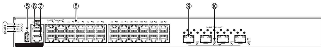
Рисунок 1-2. Передняя панель QSW-4700-28TX
