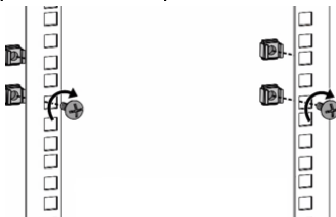
Рисунок 3-2. Установка гаек и винтов
