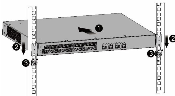
Рисунок 3-3. Затяжка винтов
