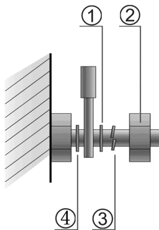
Рисунок 7-7. Крепление кабеля
