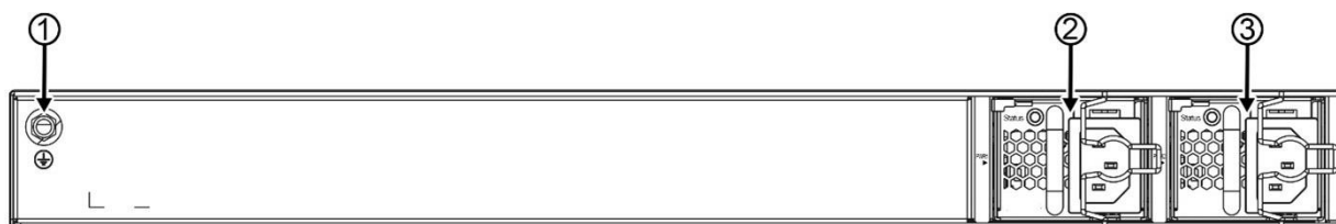
Рисунок 1-3. Задняя панель QSW-4700-28TX
