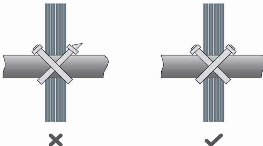
Рисунок 7-5. Стяжка кабелей
