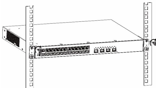
Рисунок 3-4. Затяжка остальных винтов
