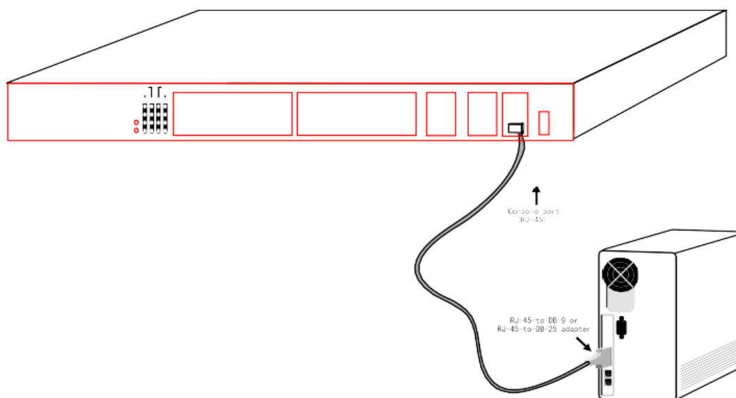
Рисунок 3-4 Подключение консольного порта QSW-5100-28FQ и компьютера
