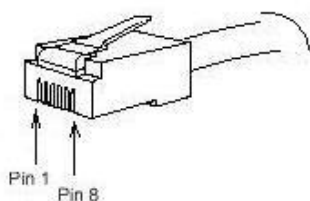
Рисунок 3-5 Разъем RJ-45 консольного порта
