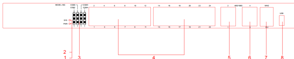
Рисунок 1-1 Лицевая панель коммутатора QSW-5100-28FQ
