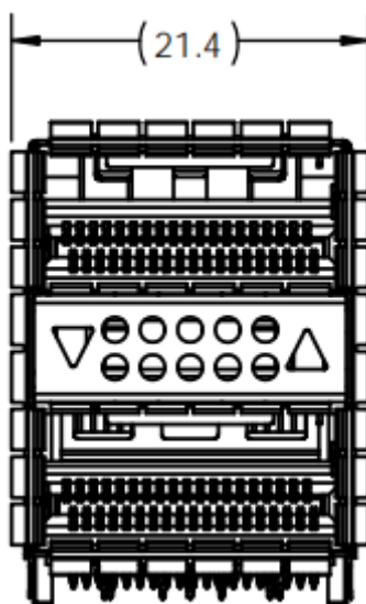
Рисунок 5-3 Индикатор порта QSFP+
