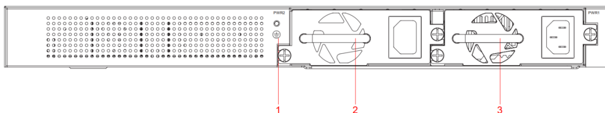
Рисунок 1-2 Задняя панель коммутатора QSW-5100-28FQ
