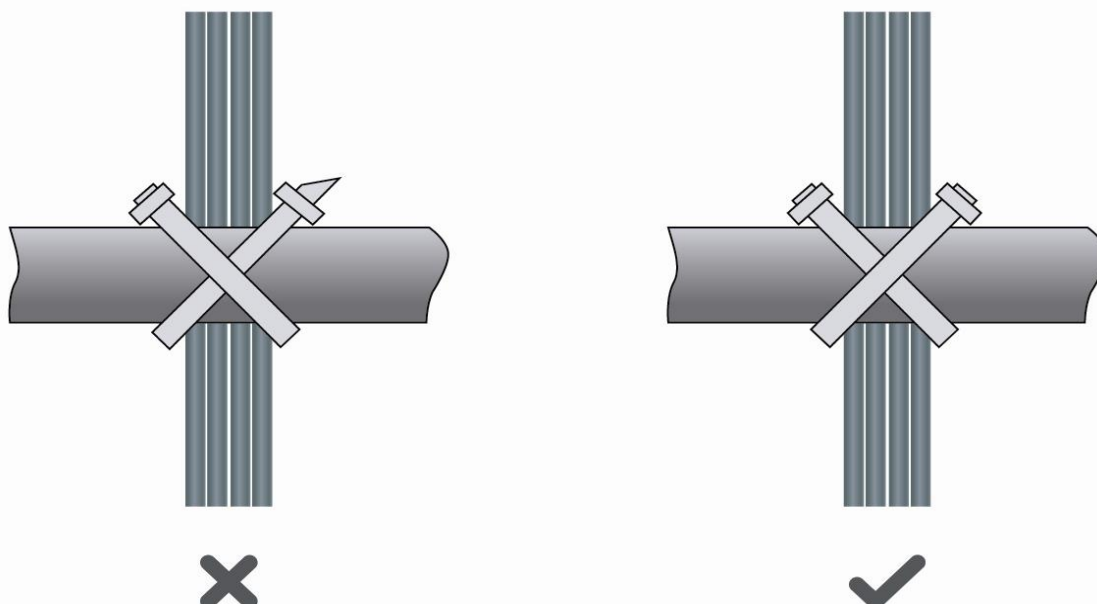
Рисунок 7-5. Стяжка кабелей
