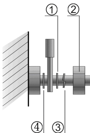
Рисунок 7-7. Крепление кабеля
