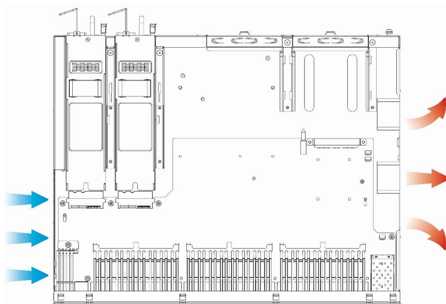
Рисунок 1-8. Направление потоков воздуха
