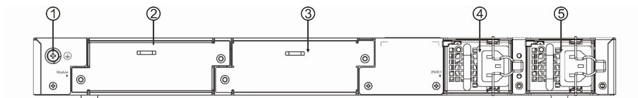
Рисунок 1-11. Задняя панель QSW-6300-32F
