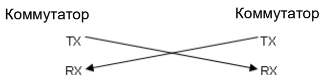
Рисунок 7-3. Подключение оптического кабеля
