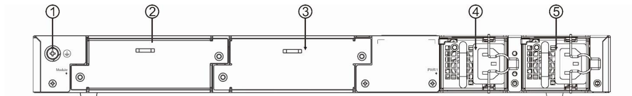
Рисунок 1-3. Задняя панель QSW-6300-32T
