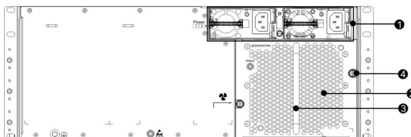
Рисунок 1-8. Задняя панель коммутатора QSW-7605
