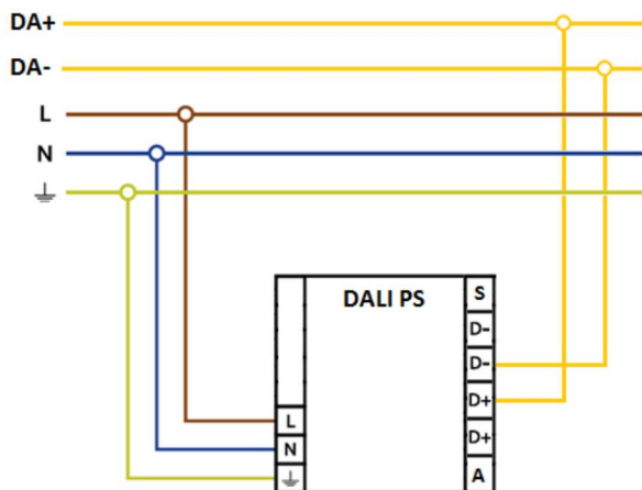
СХЕМА ПОДКЛЮЧЕНИЯ ИСТОЧНИКА ПИТАНИЯ ШИНЫ DALI
