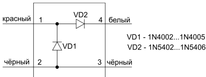
Рисунок 3. Схема модуля подключения нагрузки (МПН)
