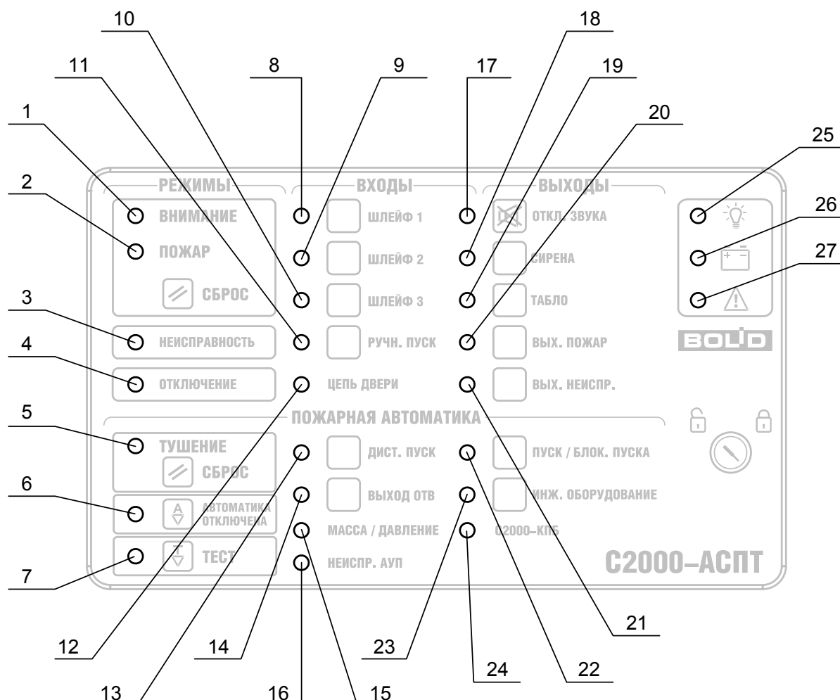
Рисунок 2.1 Расположение световых индикаторов
