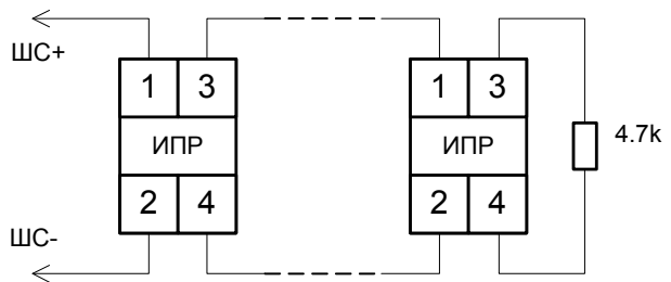
Подключение извещателей ИПР 513-3 (ИПР 513-3 исп.01, 02)
