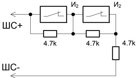
Схема подключения тепловых извещателей, тип шлейфа 3
