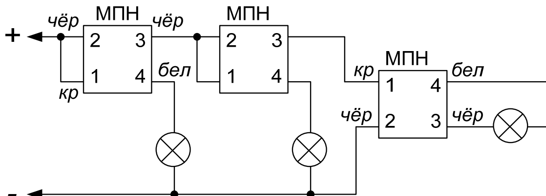
Подключение нескольких оповещателей к одному выходу прибора
