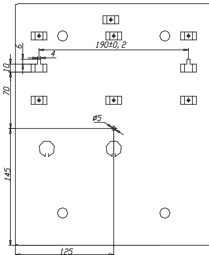
Установочные размеры
