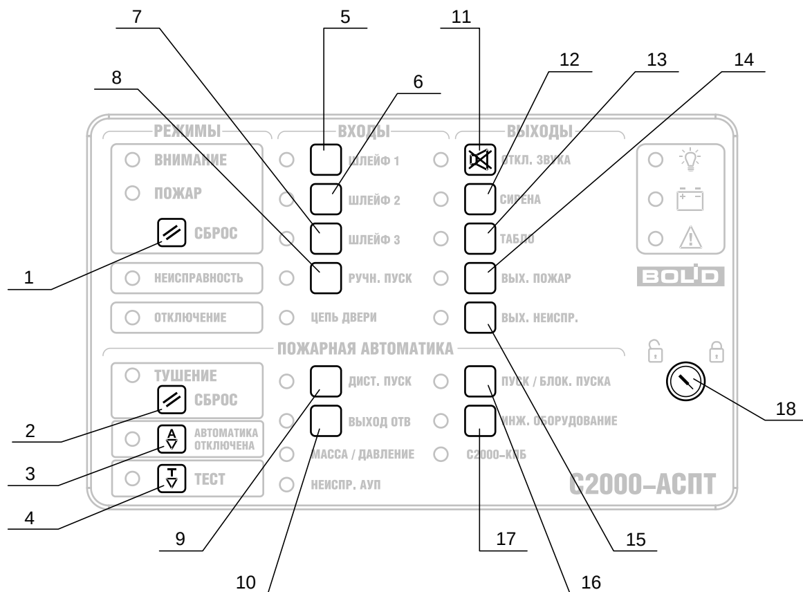
Рисунок 2. Расположение кнопок
