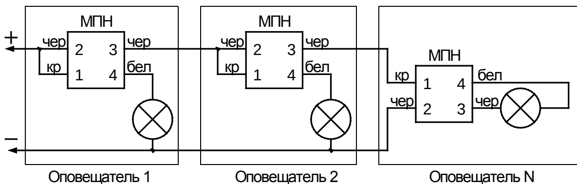
Подключение нескольких оповещателей к одному выходу блока
