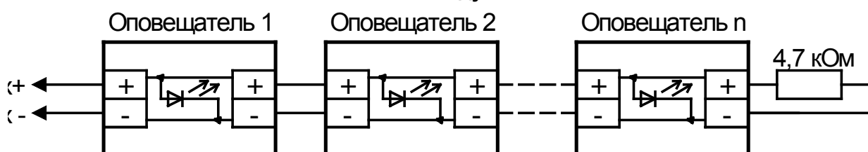
Подключение нескольких полярных оповещателей, имеющих встроенный диод, к одному выходу
