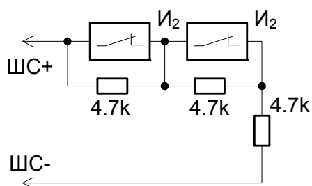
Рисунок 6. Схема подключения тепловых пожарных извещателей в шлейфы типа 3
