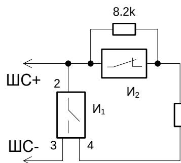
Схема подключения охранных извещателей «Фотон-СК», тип шлейфа 5
