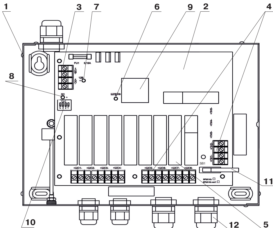
Рисунок 1 – «БРШС-Ех», вид со снятой крышкой
