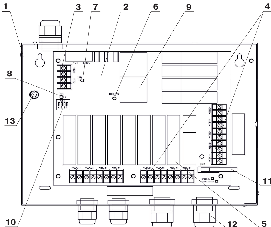
Рисунок 2 – «БРШС-Ех» исполнение 1, вид со снятой крышкой
