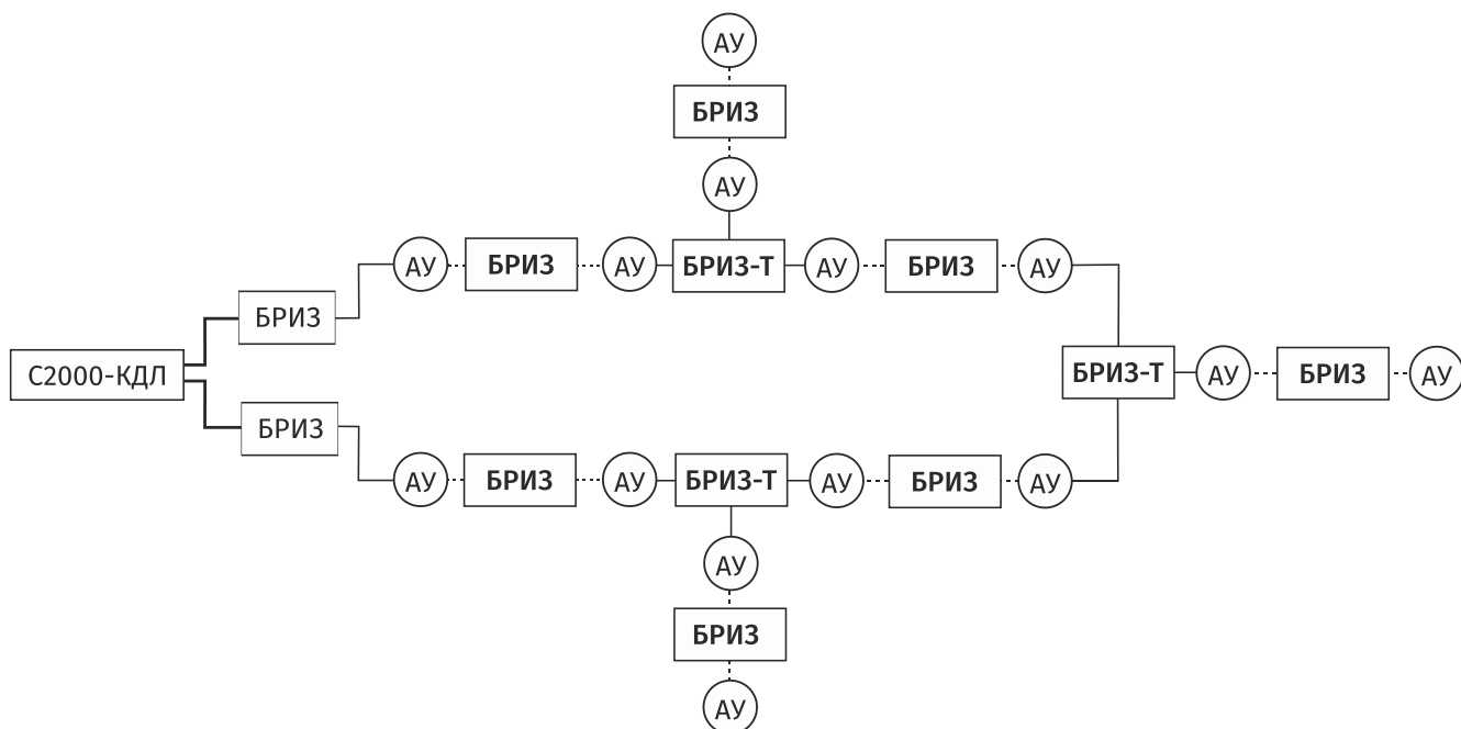
Рисунок 2.2.4.2.3 Смешанная топология
