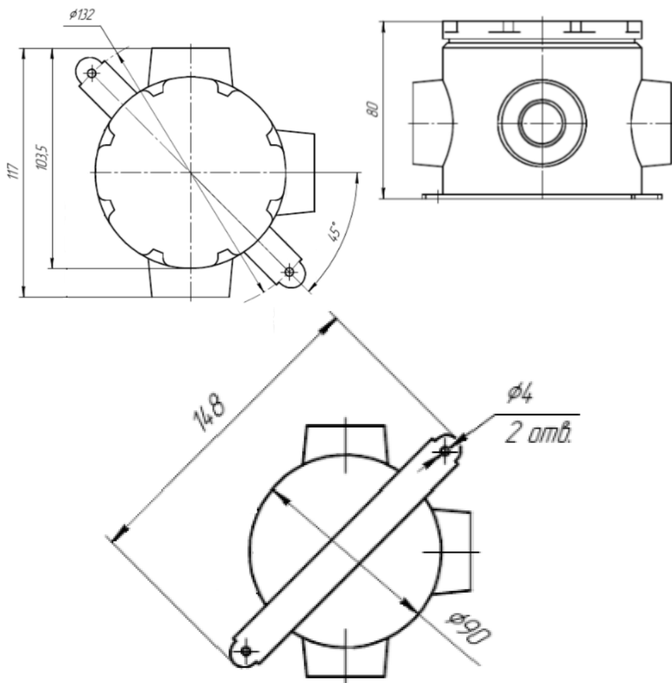
Рис.2.2.2.5 Габаритный и установочный чертежи BRI3-Exd-A-T (Вариант 2)
