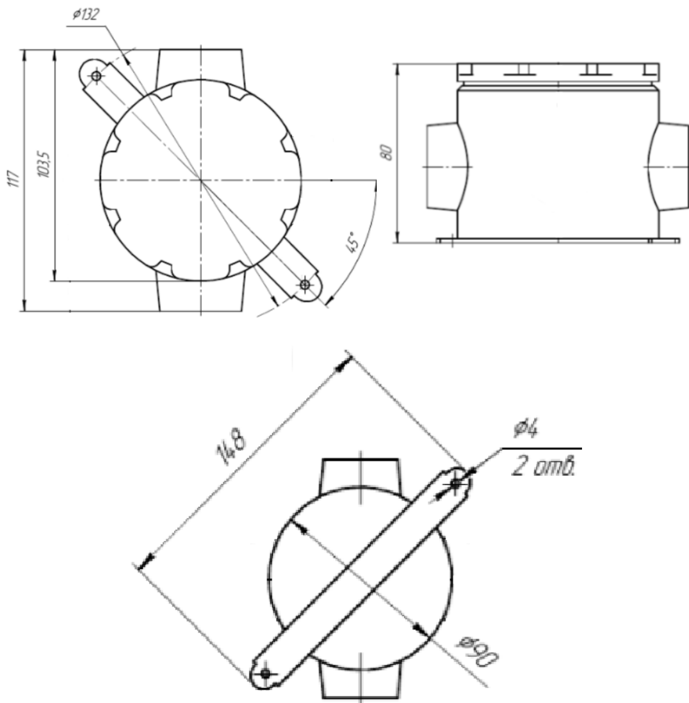
Рис.2.2.2.3 Габаритный и установочный чертежи BRI3-Exd-A (Вариант 2)
