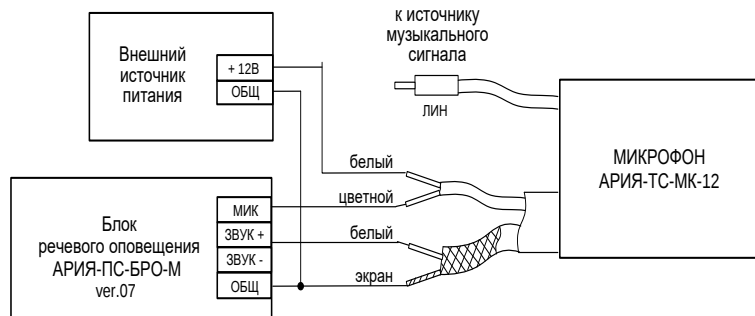
Рис.14. Схема соединений при подключении микрофона без балансного выхода.
