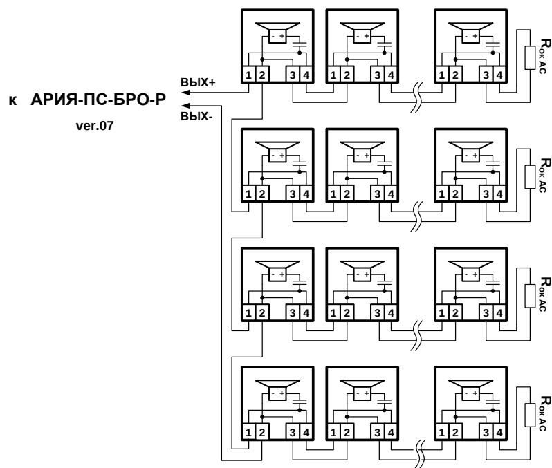
Г. Схема соединений 8, 12, 16, 20, 24, 28, 32, 36, 40, 44 и 48-ми речевых оповещателей серии АРИЯ-ПС. Номинал оконечного резистора R_{ок\ AC} = 2,4\ k\Omega \pm 5\% .
