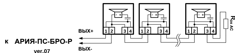
Рис.11. Схемы соединений речевых оповещателей.
