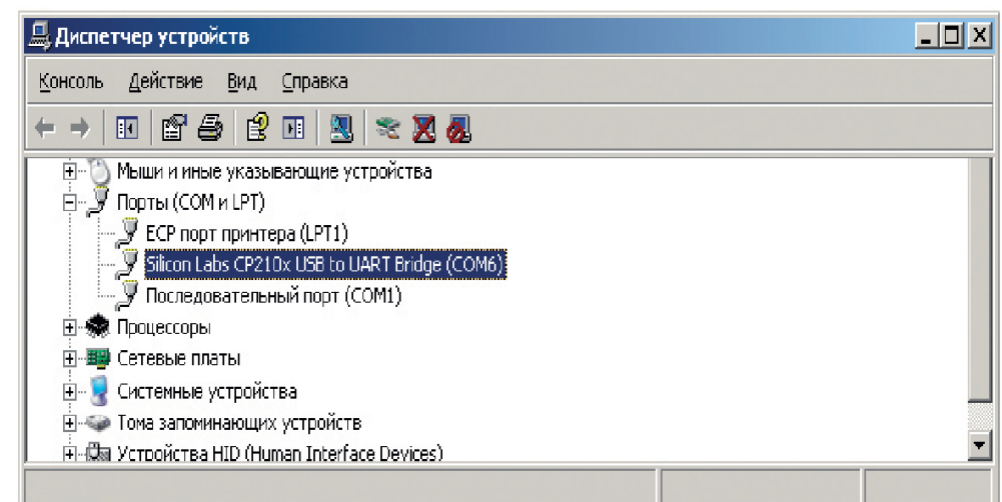
Рис.2. Диспетчер устройств.
