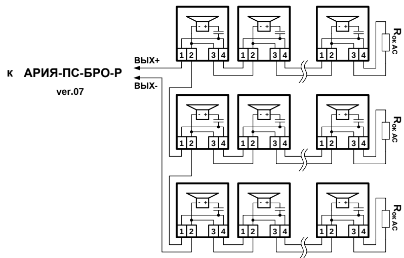
В. Схема соединений 6, 9, 12, 15, 18, 21, 24, 27, 30, 33 и 36-ти речевых оповещателей серии АРИЯ-ПС. Номинал оконечного резистора R_{ок\ AC} = 3,3\ k\Omega \pm 5\% .
