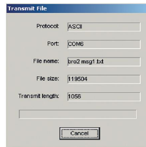
Рис. 9. Запись файла.
