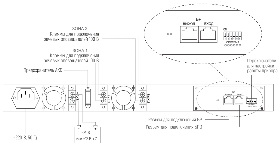
Рис. 9. Задняя панель блока расширения АРИЯ-ТС-БП-2-120
