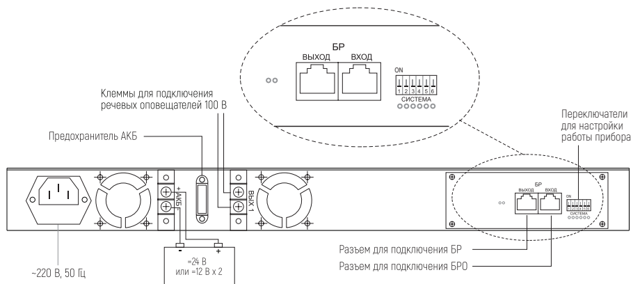
Рис. 8. Задняя панель блока расширения АРИЯ-ТС-БП-120
