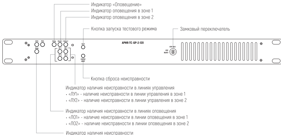
Рис. 7. Лицевая панель блока расширения АРИЯ-ТС-БП-2-120.
