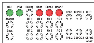
Рис. 47. Пример индикации на двухзональном БРО при трансляции сообщения с линейного входа в обе зоны оповещения
