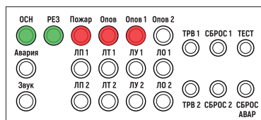
Рис. 36 Индикации на двухзональном БРО при воспроизведении сигналов оповещения по запрограммированному сценарию в зону 1
