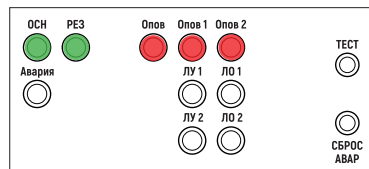
Рис. 49. Пример индикации на двухзональном БР при трансляции сообщения с линейного входа в обе зоны оповещения
