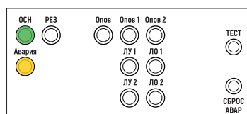
Рис. 55. Индикация на БР при отключении напряжения питания от резервного источника.
