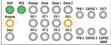
Рис. 79. Пример индикации на двухзональном БР0 после устранения неисправности в линии оповещения
