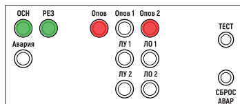
Рис. 42. Пример индикации на двухзональном БР при воспроизведении тревожного сообщения в зону 1
