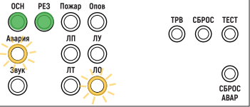
Рис. 78. Индикация на однозональном БР0 после устранения неисправности в линии оповещения
