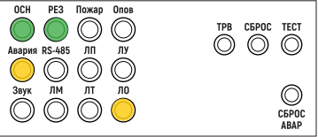
Рис. 74. Индикация на однозональном БР0 при неисправности в линии оповещения
