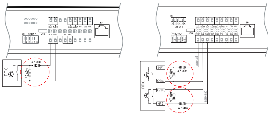
Рис. 10. Подключение ППК. Контроль целостности линий связи
