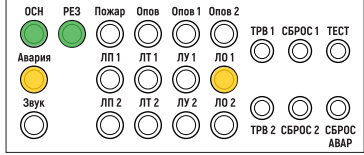
Рис. 75. Пример индикации на двухзональном БР0 при неисправности в линии оповещения в зоне 1
