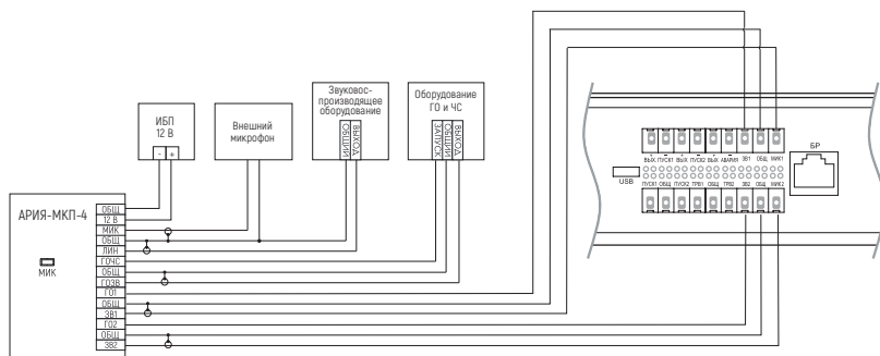
Рис. 45. Схема подключения микрофонной панели АРИЯ-МКП-4
