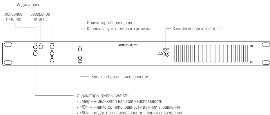
Рис.6. Лицевая панель блока расширения АРИА-ТС-БР-120.
