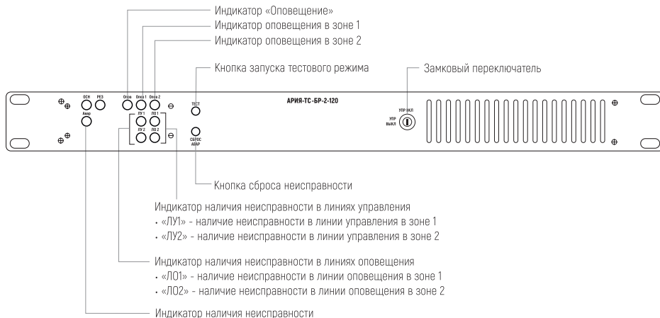
Рис. 7. Лицевая панель блока расширения АРИА-ТС-БР-2-120.
