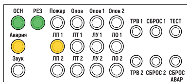
Рис. 59. Пример индикации на двухзональном БРО при неисправности в зоне 1 в линии связи между изделием и ППК
