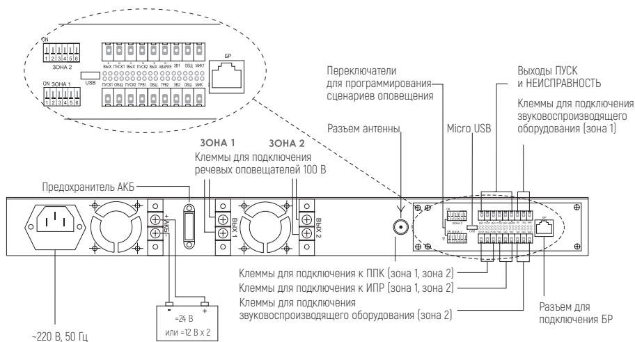
Рис. 5. Задняя панель блока речевого оповещения АРИЯ-ТС-БРО-2-120
