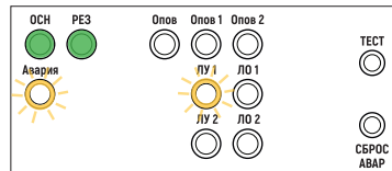
Рис. 73. Пример индикации на двухзональном БР после устранения неисправности в линии управления в зоне 1.
