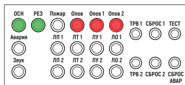
Рис. 47 Пример индикации на двухзональном БРО при трансляции сообщения с линейного входа в обе зоны оповещения
