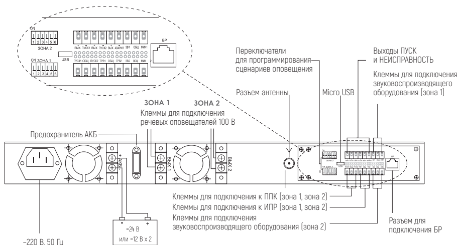
Рис. 5. Задняя панель блока речевого оповещения АРИЯ-ТС-БРО-2-120
