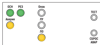
Рис. 19. Индикация режима «Неисправность» на однозональном и двухзональном БР
