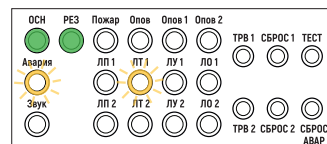
Рис. 65. Индикация на двухзональном БРО после устранения неисправности
