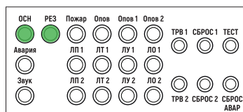
Рис. 28. Индикация режима «Дежурный» на двухзональном БРО
