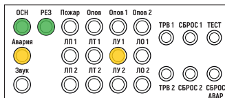
Рис. 67. Пример индикации на двухзональном БРО при неисправности в линии управления в зоне 1.
