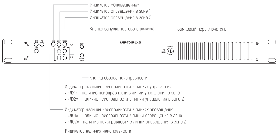
Рис. 7. Лицевая панель блока расширения АРИЯ-ТС-БР-2-120.
