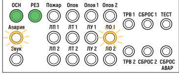
Рис. 79. Пример индикации на двухзональном БРО после устранения неисправности в линии оповещения
