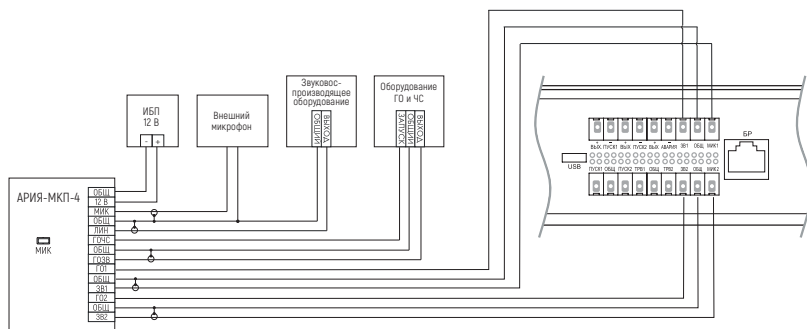
Рис. 45. Схема подключения микрофонной панели АРИЯ-МКП-4
