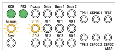
Рис. 61. Индикации после устранения неисправности в зоне 1 в двухзональном БРО
