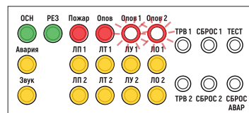
Рис. 85. Пример индикации при отсутствии в памяти двухзонального БРО тестового сообщения для зоны 1
