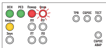
Рис. 82. Индикация при отсутствии в памяти однозонального БРО сообщения для персонала или тревожного сообщения
