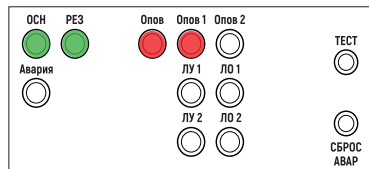
Рис. 38 Индикация на двухзональном БР при воспроизведении сигналов оповещения по запрограммированному сценарию в зону 1
