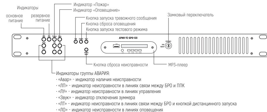
Рис. 2. Лицевая панель блока речевого оповещения АРИЯ-ТС-БРО-120.
