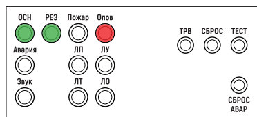
Рис. 46. Индикация на однозональном БРО при трансляции сообщения с линейного входа
