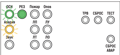
Рис. 52. Индикации на БРО после устранения неисправности.
