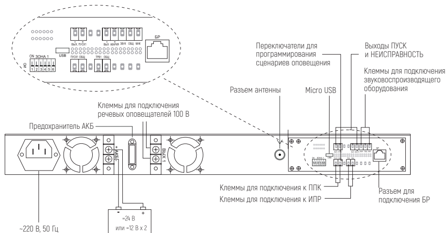
Рис. 4. Задняя панель блока речевого оповещения АРИЯ-ТС-БРО-120
