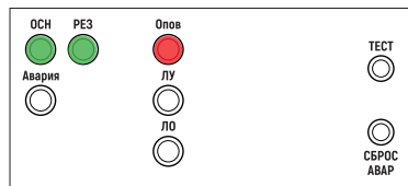
Рис. 48. Индикация на однозональном БРО при трансляции сообщения с линейного входа
