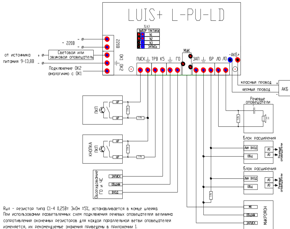
Рисунок 2. Схема внешних соединений прибора «LUIS+ L-PU-LD»
