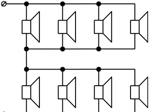
Подключение восьми акустических оповещателей Zн=4 Ом, Рн=3Вт; Рвых<3Вт/оповещатель – рис.3
