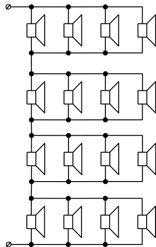
Подключение шестнадцати акустических оповещателей Z_{ли}=4\text{ Ом} , P_{ли}=3\text{ Вт} ; P_{выс}\approx 0,9\text{ Вт/оповещатель} – рис. 8
