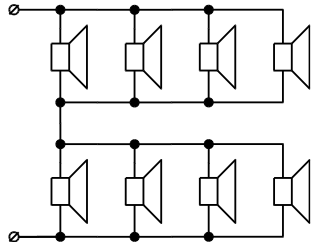
Подключение восьми акустических оповещателей Z_{ли}=8\text{ Ом} , P_{ли}=3\text{ Вт} ; P_{выс}\approx 1,85\text{ Вт/оповещатель} – рис. 6
