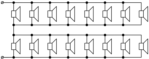
Подключение шестнадцати акустических оповещателей Zн=8 Ом, Рн=3Вт; Рвых<1,5 Вт/оповещатель – рис.4
