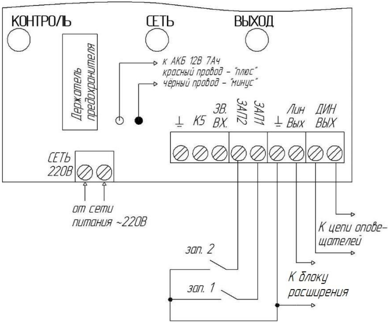
Схема внешних соединений прибора «LUIS+ L-PU-LM исп. light», рис.1
