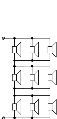
Подключение девяти акустических оповещателей Z_{ли}=4\text{ Ом} , P_{ли}=3\text{ Вт} ; P_{выс}\approx 1,65\text{ Вт/оповещатель} – рис. 7
