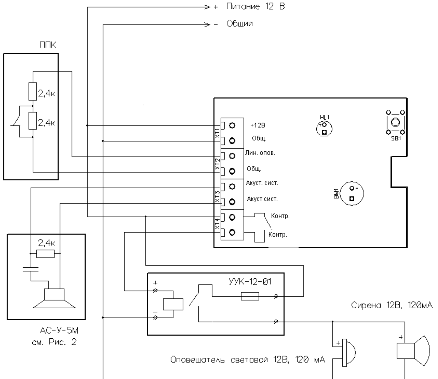
Рисунок 1. Типовая схема подключения
