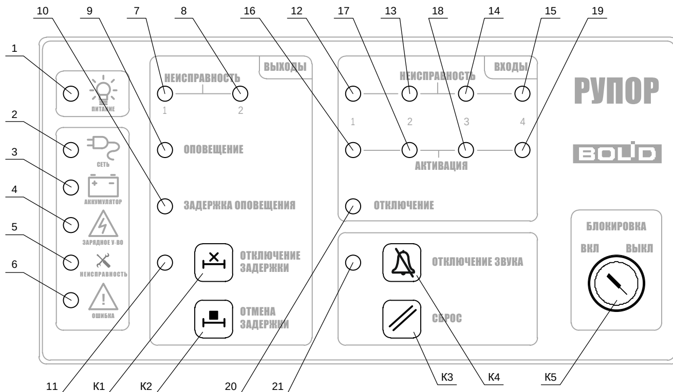
Рисунок 1. Органы управления и индикации прибора
