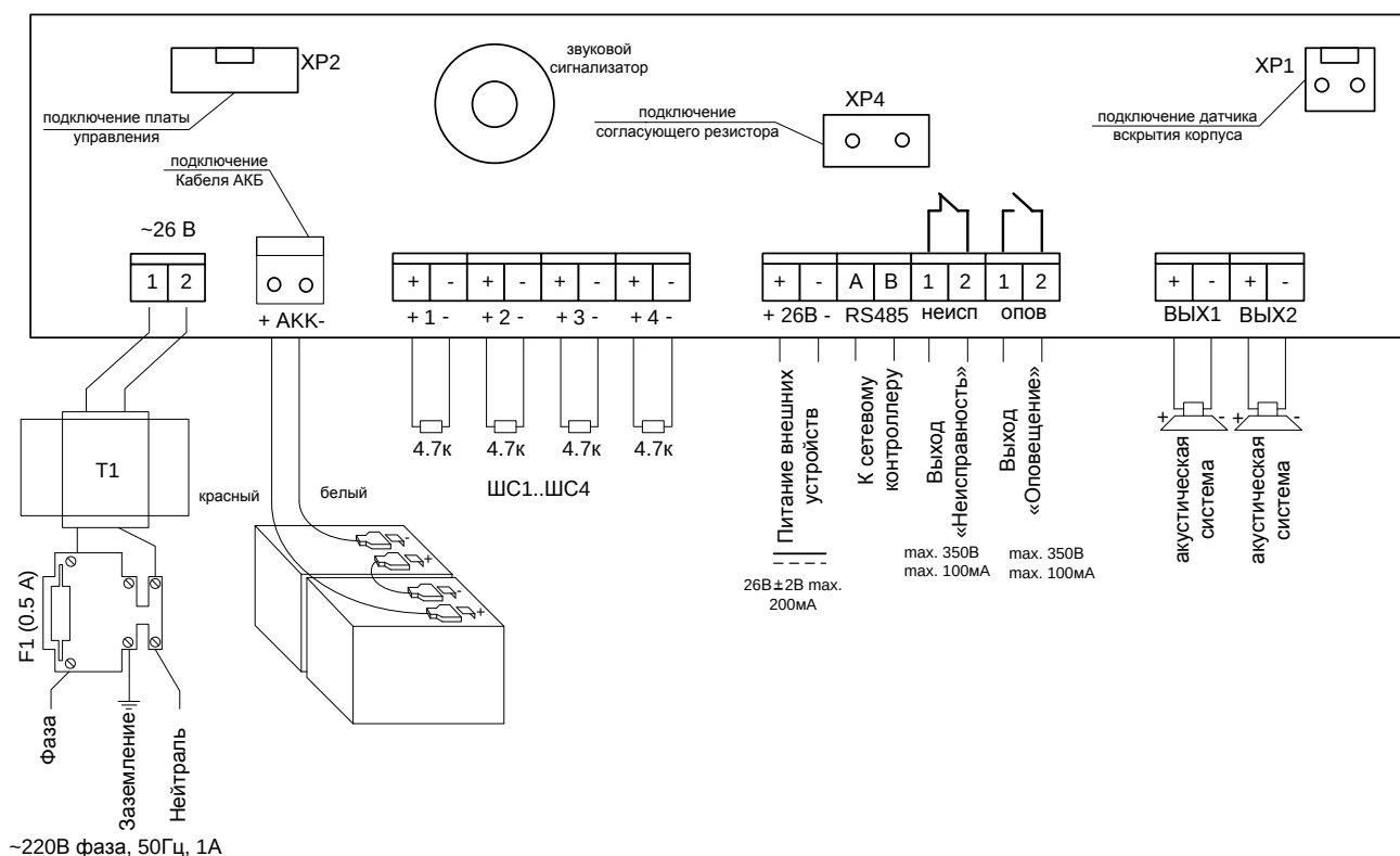
Рисунок 5. Схема подключения прибора
