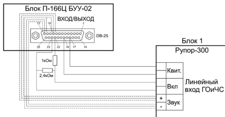
Рисунок 2.5. Схема подключения блока управления П-166Ц БУУ-02.
