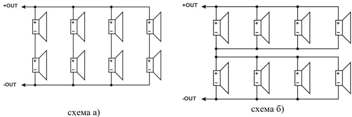
Рис. А4. Вариант 1 подключения РО
