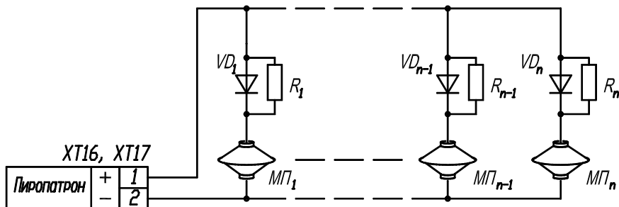
Рис.2.8. Подключение исполнительных устройств
