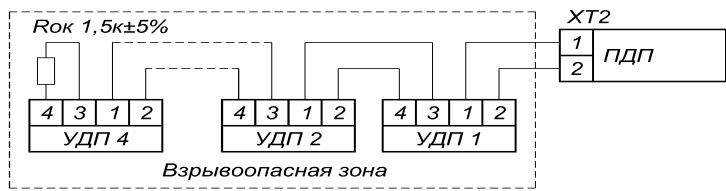
Рис.2.3. Подключение УДП.
