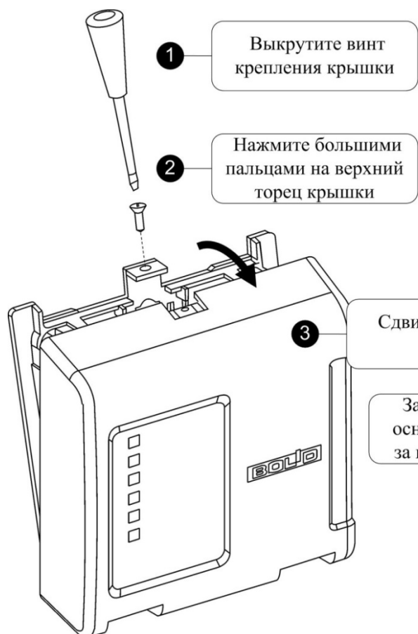
Рисунок 2.2.2 – Снятие крышки корпуса блока
