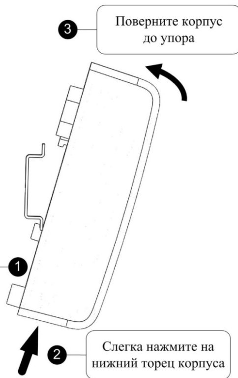
Рисунок 2.2.3 – Схема установки блока на DIN рейку.
