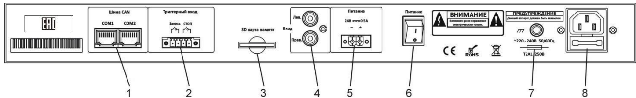
Рис. 3.3. Задняя панель блока записи сообщений LPA-EVA-RC
