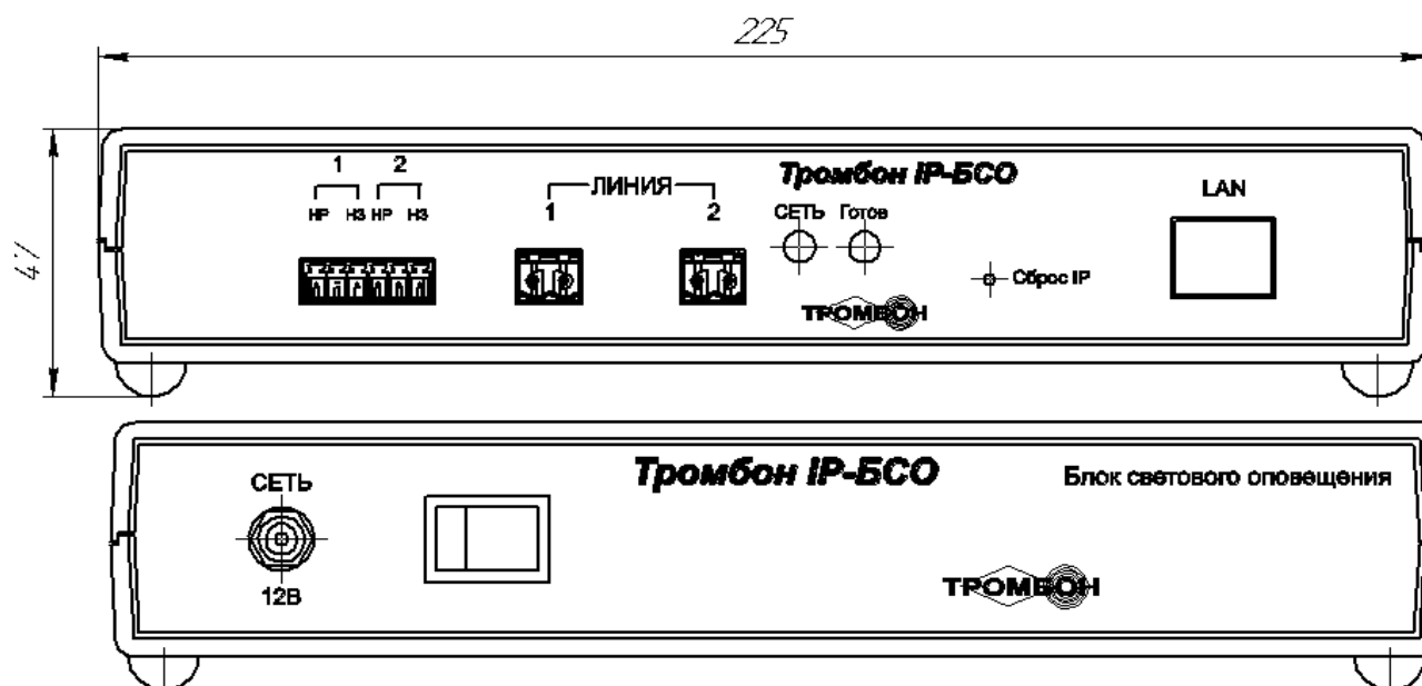
Рисунок 1-Общий вид
