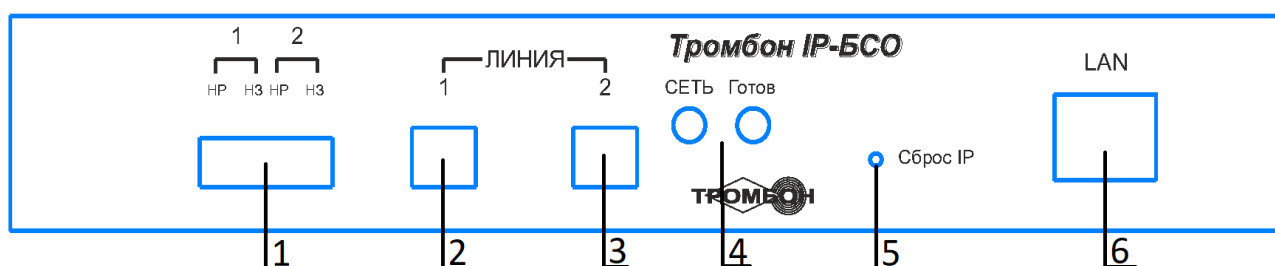
Рисунок 2-Вид спереди
