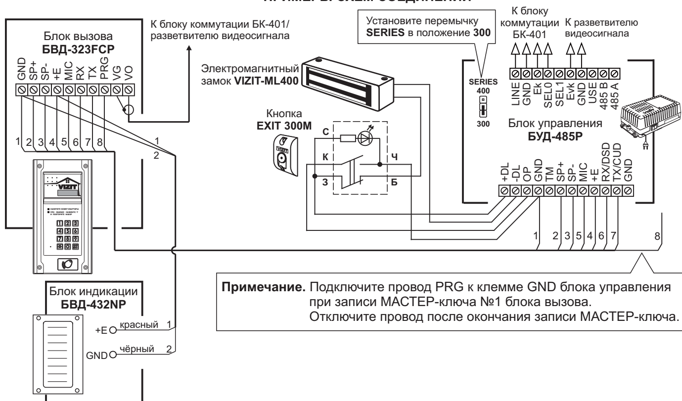
Рисунок 1 - Схема соединений блока вызова БВД-323FCР с блоком управления БУД-485Р , блоком индикации БВД-432NP , электромагнитным замком VIZIT-ML400 и кнопкой EXIT 300M
