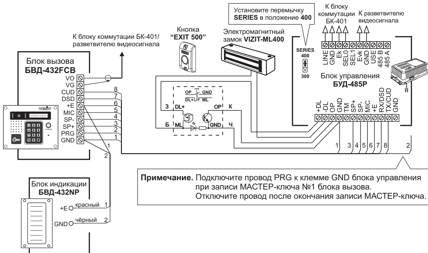
Рисунок 3 - Схема соединений блока вызова БВД-432FCB с блоком управления БУД-485Р , блоком индикации БВД-432NP , электромагнитным замком VIZIT-ML400 и кнопкой "EXIT 500"
